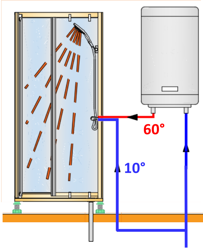
Installation Classique
